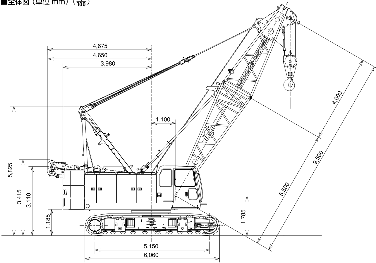
■全体図 (単位 mm) ( \frac{1}{100} )
