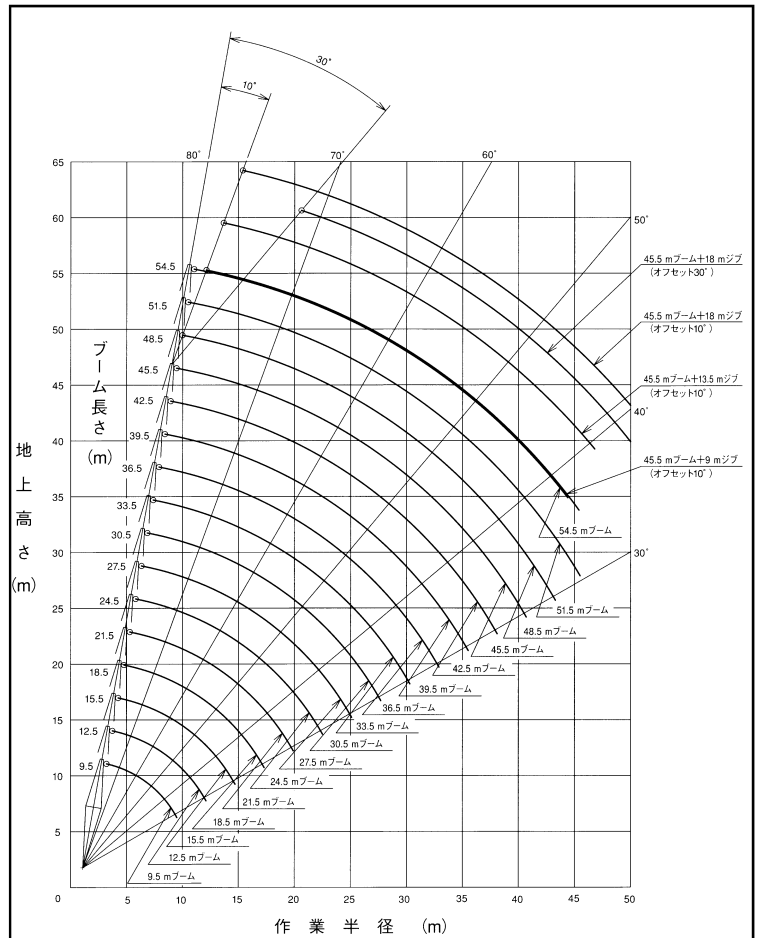
■作業範囲図
